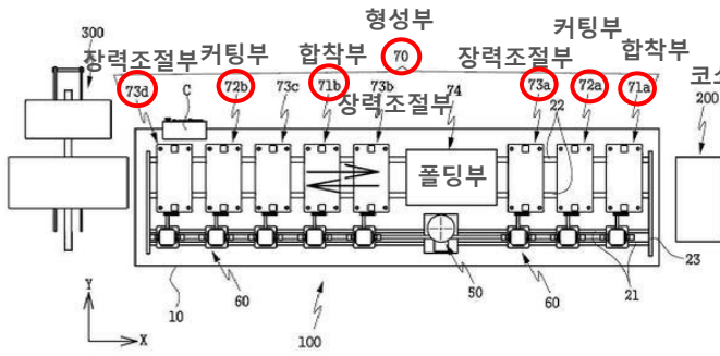
<마스크 본체 형성 장치>
